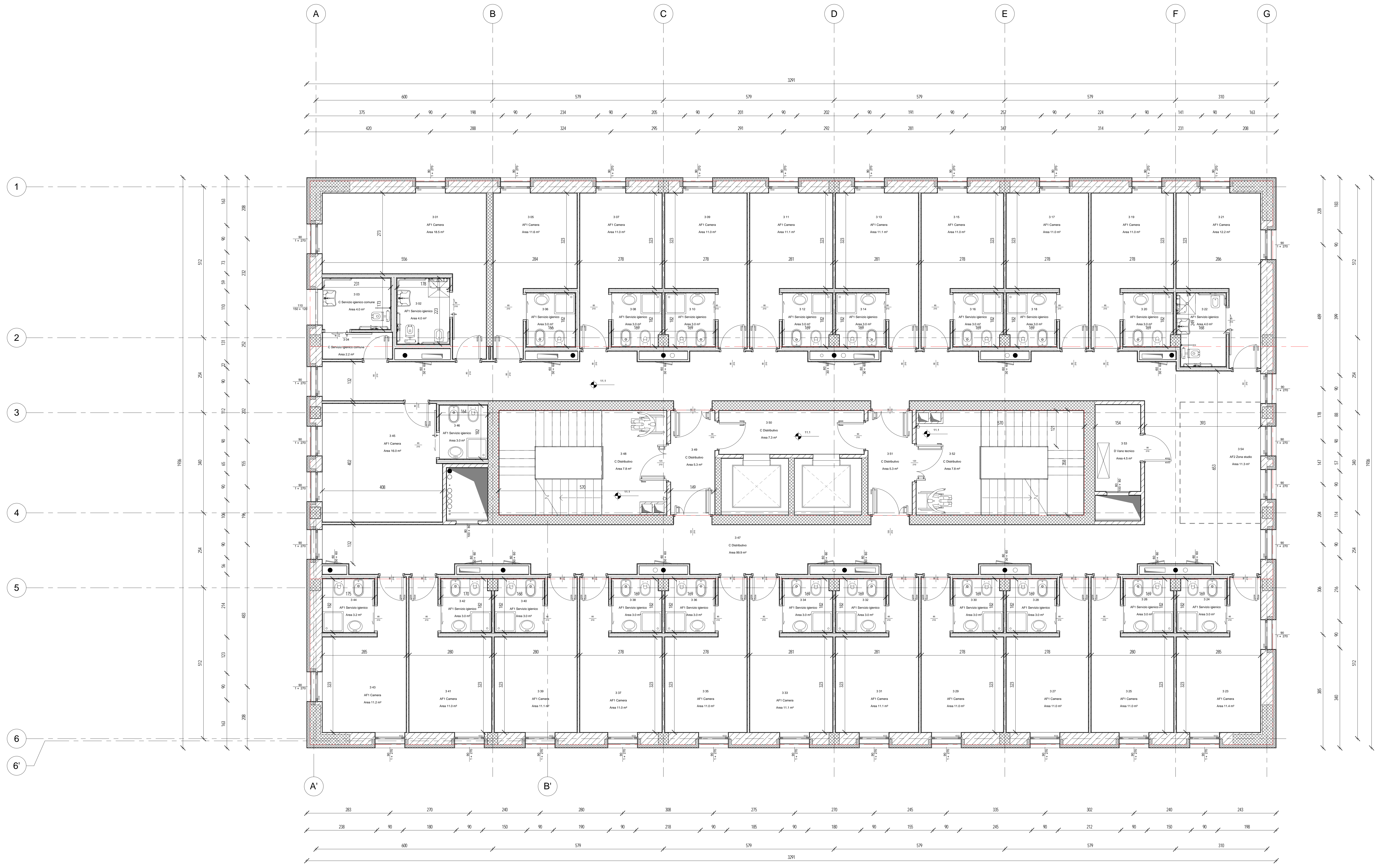
Piano terzo Scala: 1:50
