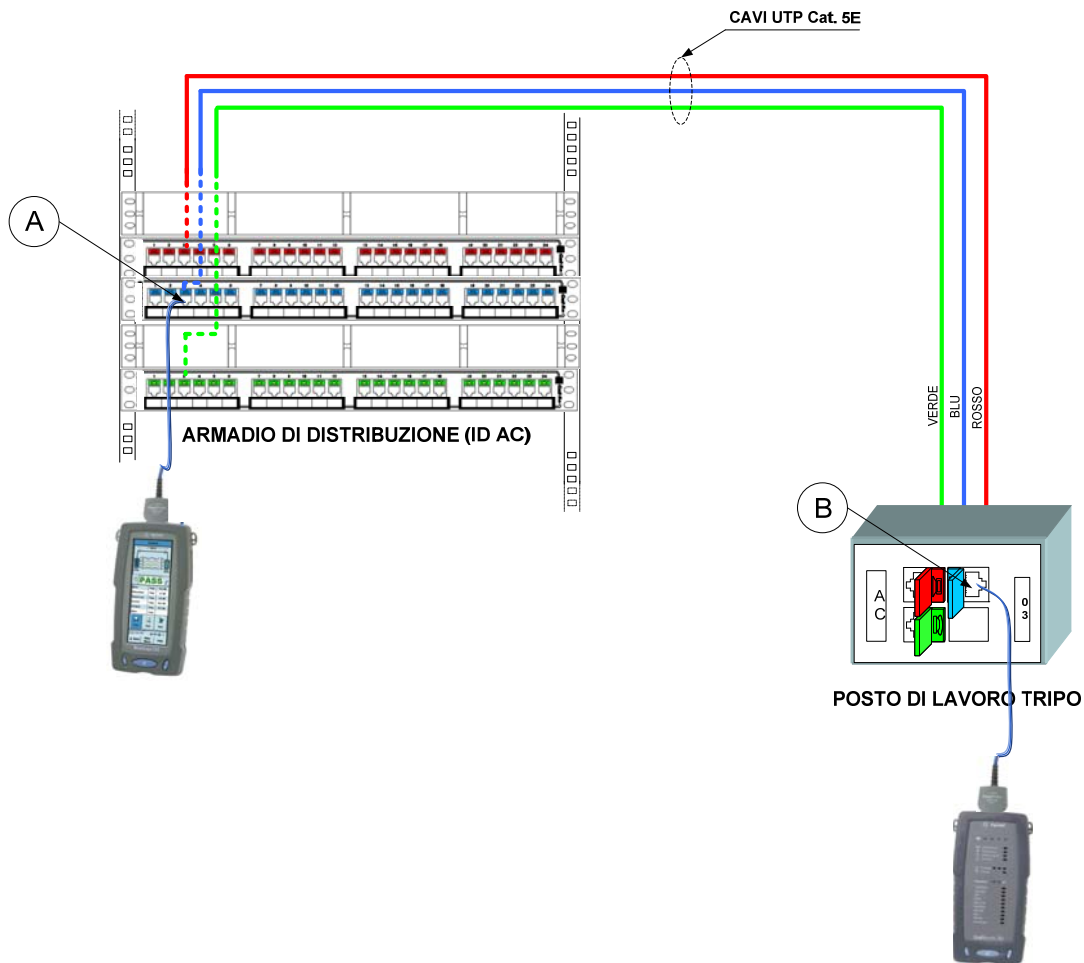
Figura 17 – Il permanent Link A-B
