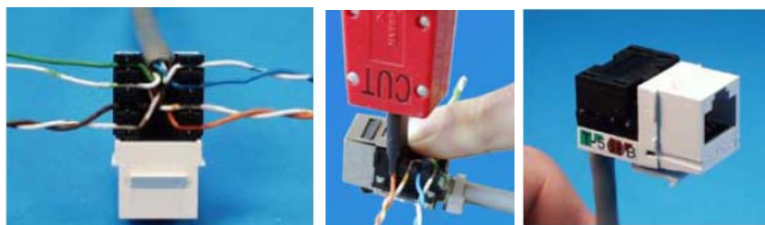
Figura 7 – Esempi di prese telematiche RJ45 e modalità di connettorizzazione
