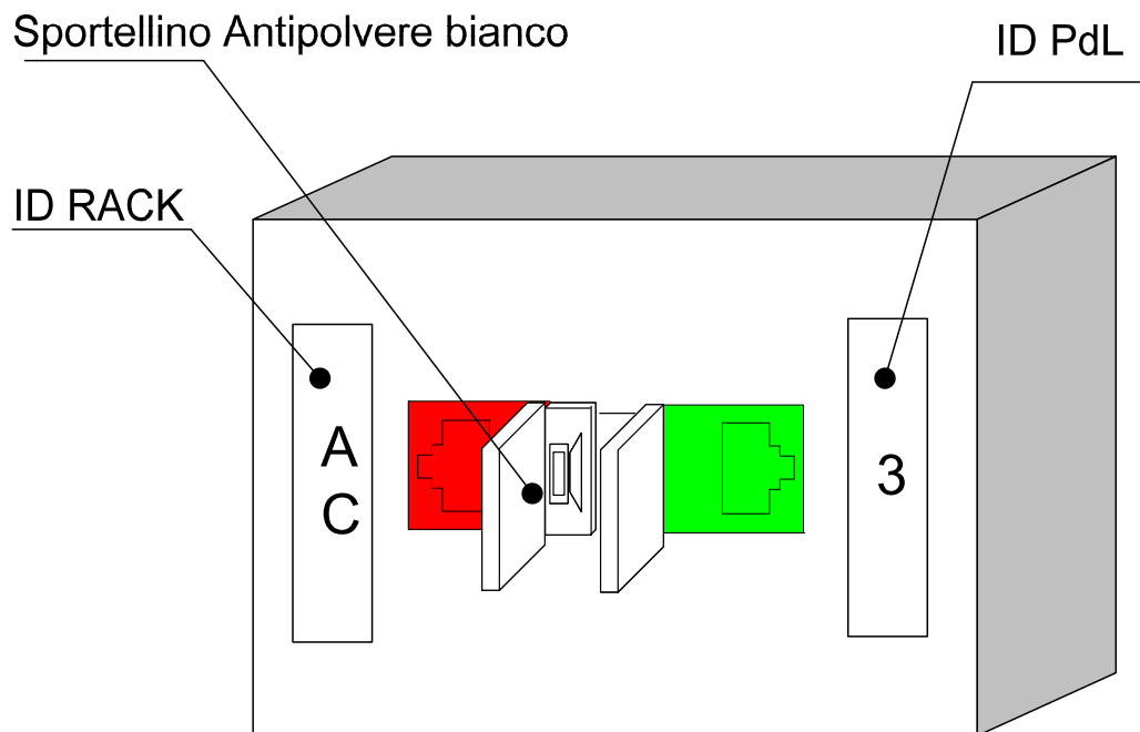
Figura 4 – Esempio di PdL Doppio
