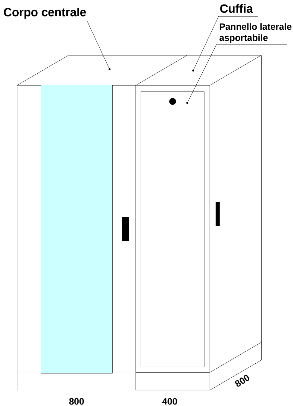
Figura 14 – Armadio di permutazione con cuffia laterale
