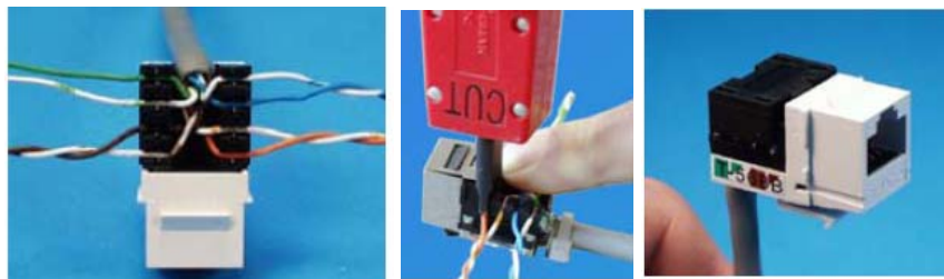
Figura 9 – Esempio di connettorizzazione mediante impact tool
